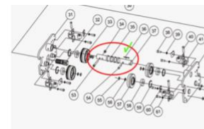
Вал для каретки на ТЭЦ 3т на двутавр шириной до 178мм
