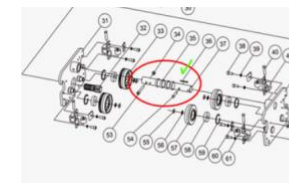
Вал удлиненный для каретки на ТЭЦ 500кг на двутавр шириной 300мм
