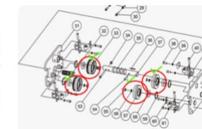
Колёса грузовые для электро каретки 500кг комплект
