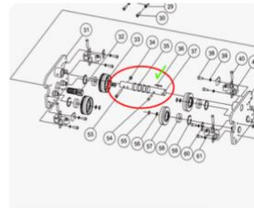
Вал для каретки на ТЭЦ 500кг на двутавр шириной до 178мм
