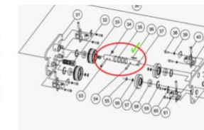
Вал удлиненный для каретки на ТЭЦ 1т на двутавр шириной 300мм
