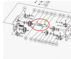
Вал для каретки на ТЭЦ 1т на двутавр шириной до 178мм
