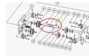
Вал для каретки на ТЭЦ 5т на двутавр шириной до 178мм
