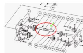
Вал удлиненный для каретки на ТЭЦ 2т на двутавр шириной 300мм
