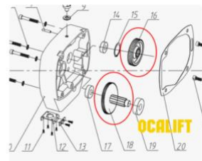
Редукторная пара 00501
