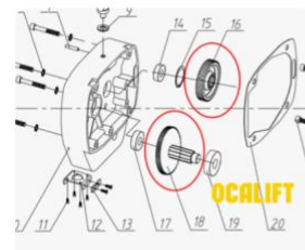
Редукторная пара 02501/0301/0502
