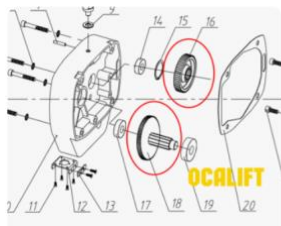
Редукторная пара 0101/0202
