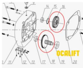
Редукторная пара 0201/0302
